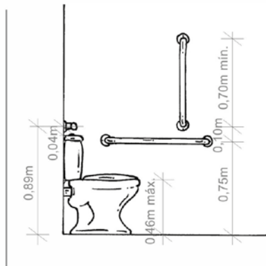
VISTA LATERAL
